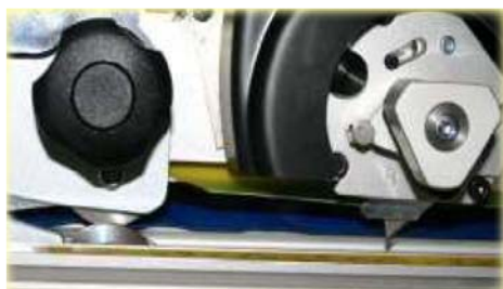
Les 2 outils sont présentés en position basse. Un seul outil est engagé lors de l'utilisation.
